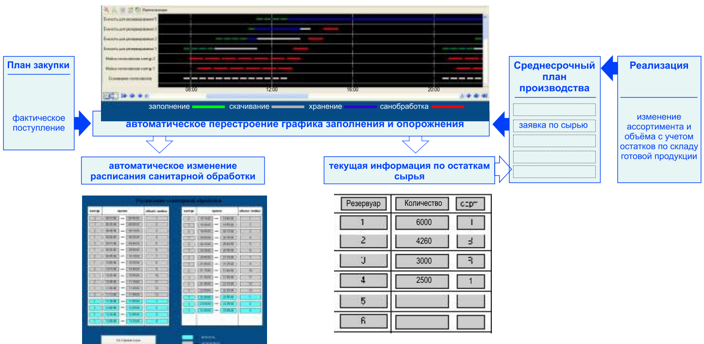
График заполнения и опорожнения резервуаров хранения
